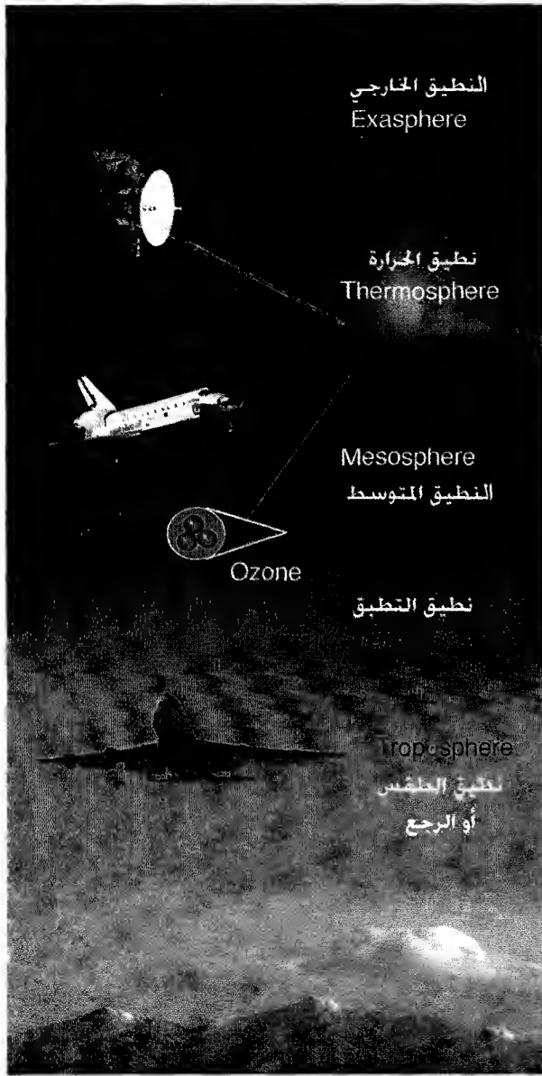
رسم تخطيطي لتكوين الغلاف الغازي للأرض
